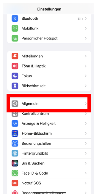
Abbildung 1: iOS Geräteeinstellungen
