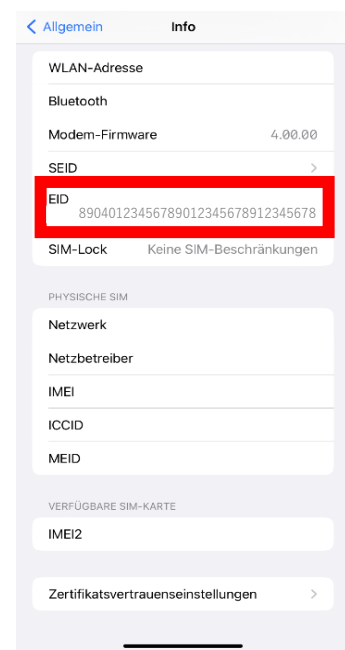
Abbildung 3: Deine eID
